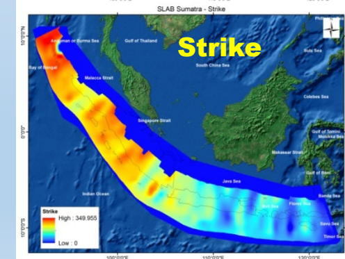
(subduction zone geometry)
